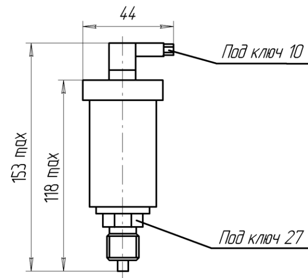
Рис. 2.2 Преобразователь давления ПДТВХ-1 с разъёмом по DIN 43650.
