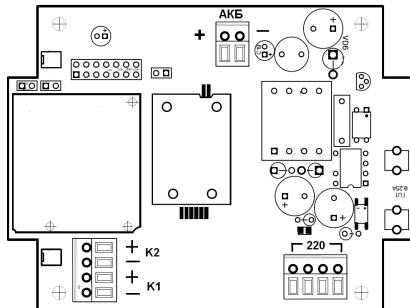
Рис. 7.1 Схема клеммников счетчика
