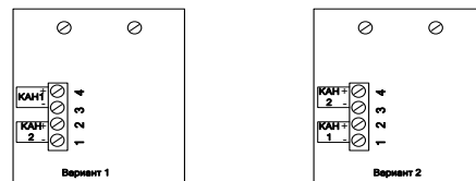
Рис. 7.2 Схема клемников передающего модуля (вариант 2 исполнение «Н»)
